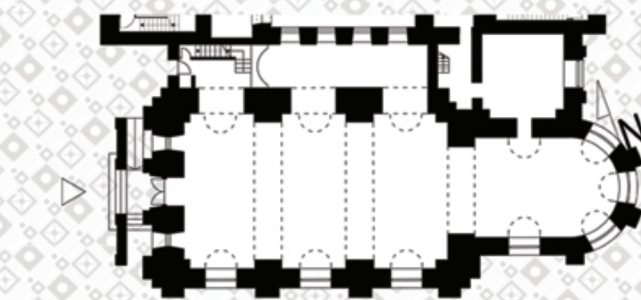
ПЛАН НИЖНЕГО ЭТАЖА
