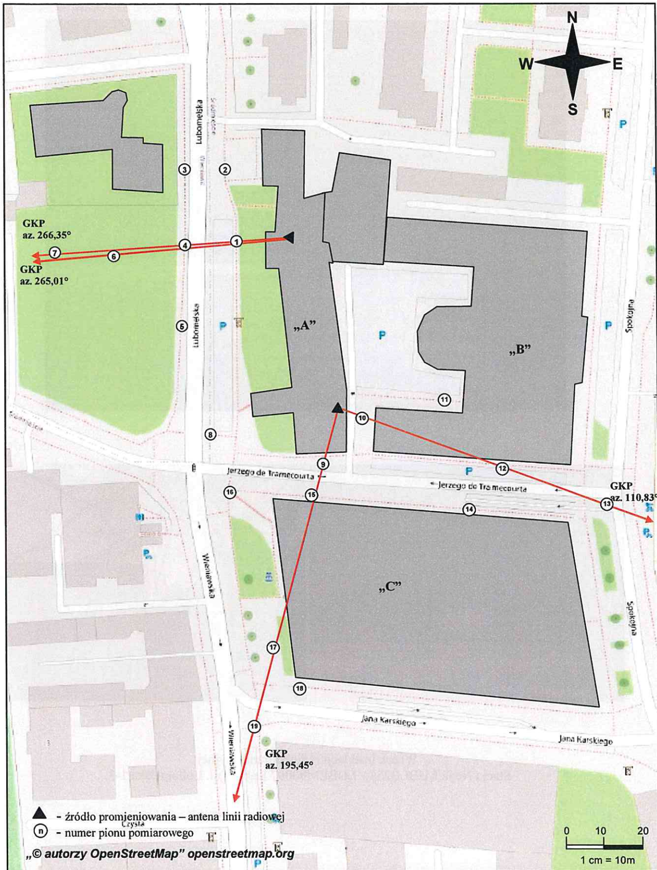
Rys. 1. Usytuowanie punktów i pionów pomiarowych w otoczeniu instalacji radiokomunikacyjnej Stacja Netia LUBLB251-LUBLM00007 Lublin, ul. Lubomelska 1-3
