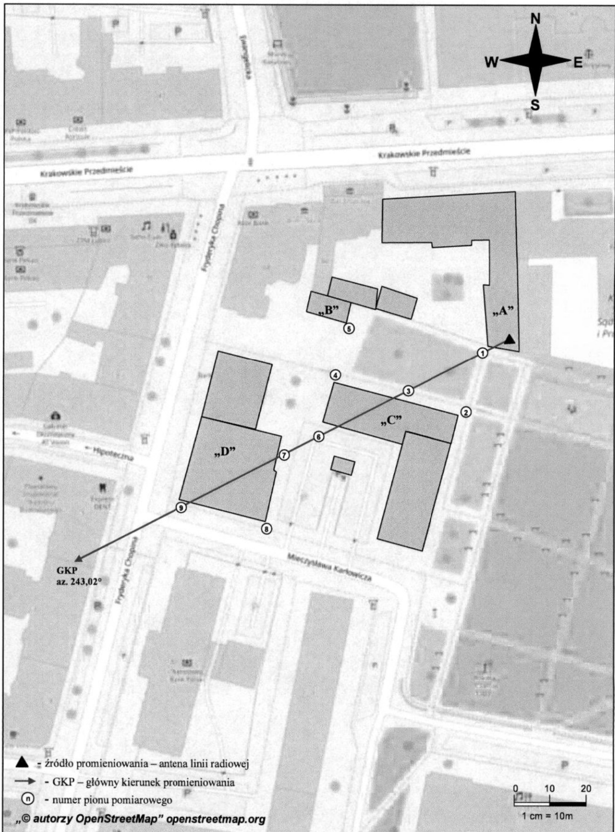
Rys. 1. Usytuowanie punktów i pionów pomiarowych w otoczeniu instalacji radiokomunikacyjnej Stacja Netia LUBLB631-LUBLM00280 Lublin, ul. Krakowskie Przedmieście 64
