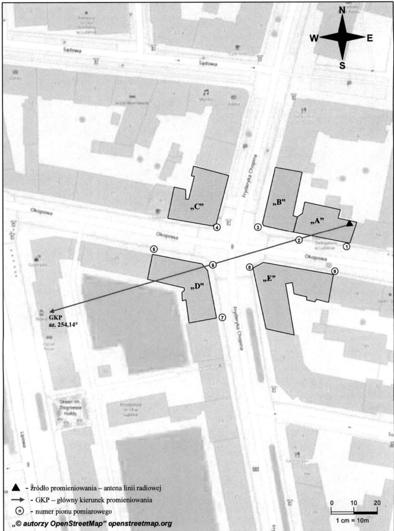
Rys. 1. Usytuowanie punktów i pionów pomiarowych w otoczeniu instalacji radiokomunikacyjnej Stacja Netia LUBLB318-LUBLM00244 Lublin, ul. Okopowa 7
