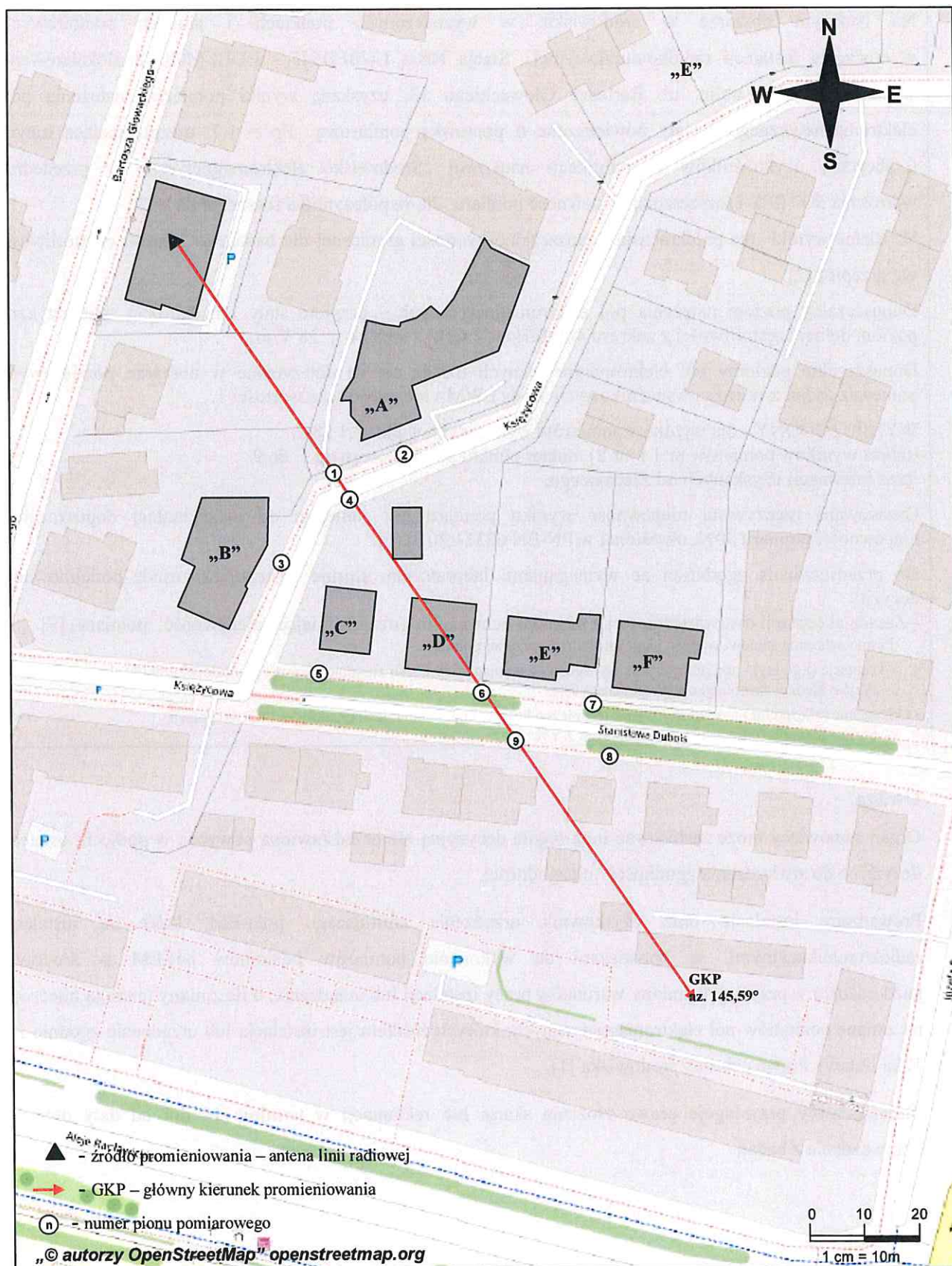
Rys. 1. Usytuowanie punktów i pionów pomiarowych w otoczeniu instalacji radiokomunikacyjnej Stacja Netia LUBLB547-LUBLM00278 Lublin, ul. Bartosza Głowackiego 13
