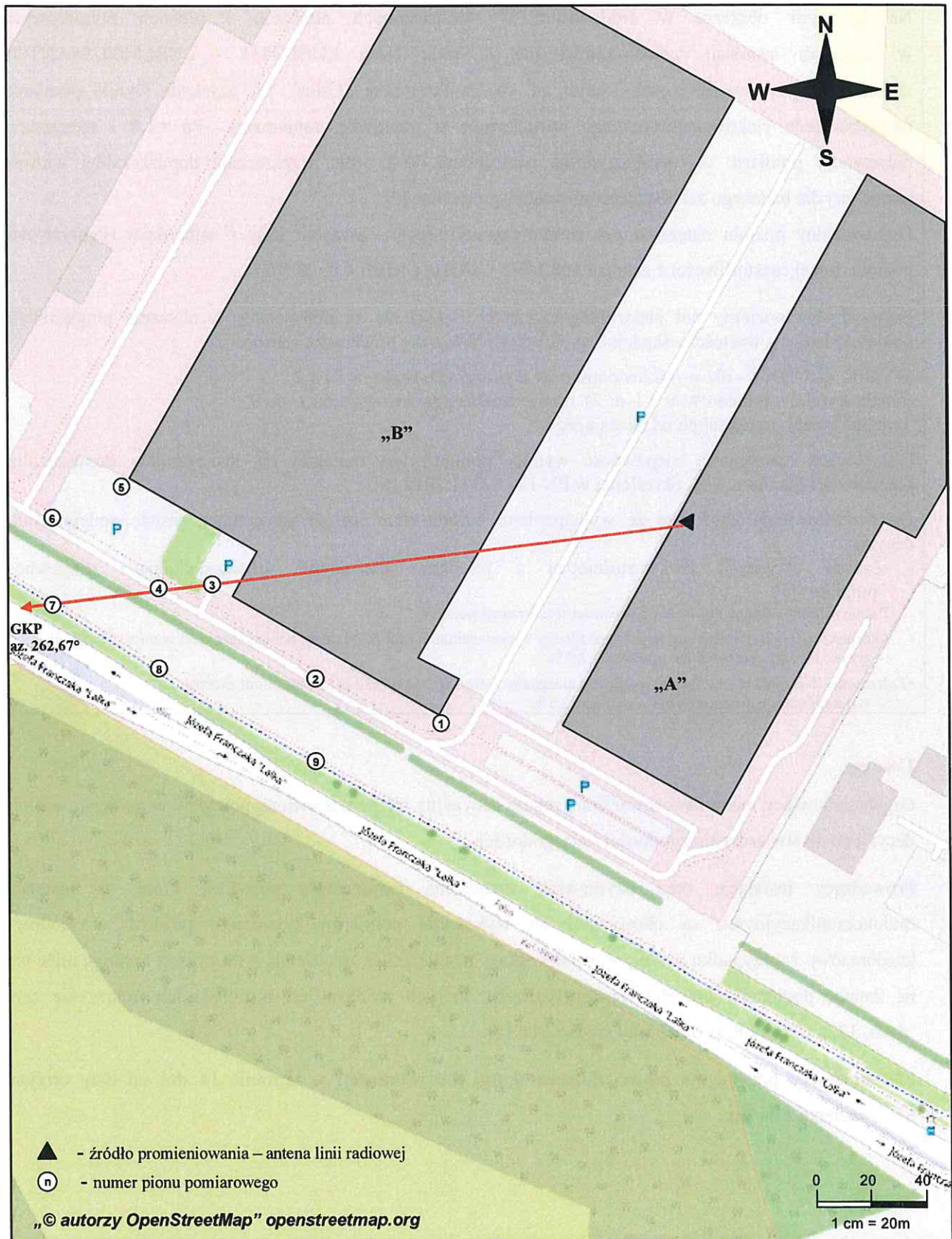
Rys. 1. Usytuowanie punktów i pionów pomiarowych w otoczeniu instalacji radiokomunikacyjnej Stacja Netia LUBLB831-LUBLM00296ANT001 Lublin, ul. Józefa Franczaka „Lalka” 18
