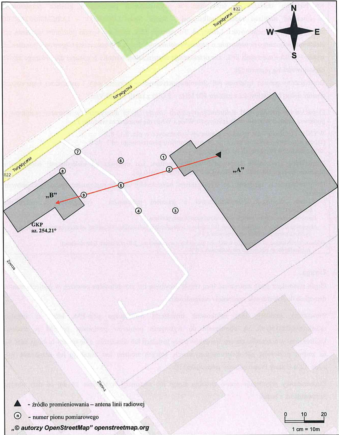
Rys. 1. Usytuowanie punktów i pionów pomiarowych w otoczeniu instalacji radiokomunikacyjnej Stacja Netia LUBLB351-LUBLM00257ANT003 Lublin, ul. Turystyczna 11A
